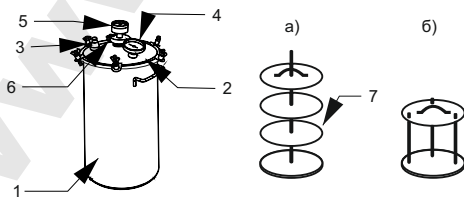
Рисунок 1. Общее устройство автоклава.
