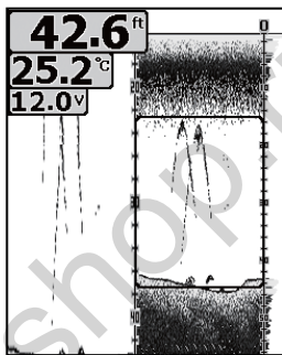
ЭКРАН ЭХОЛОТА С МАСШТАБИРОВАНИЕМ (83 КГц)
